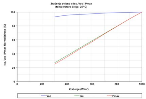
ZRAČENJE
