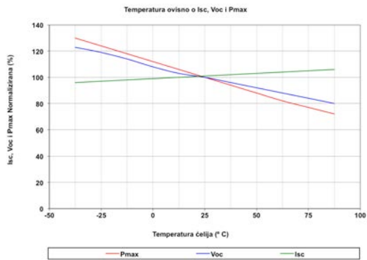
TEMPERATURA
