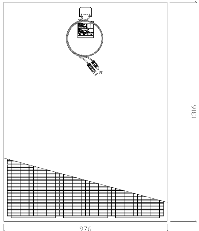
VUE ARRIÈRE
