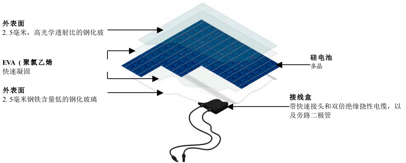
结构详图
