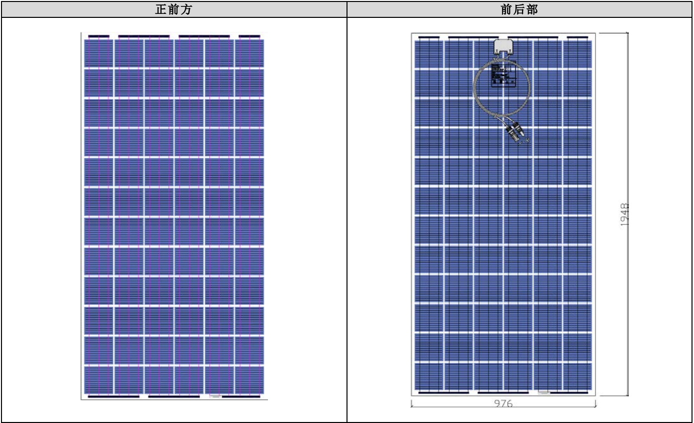
结构详图
